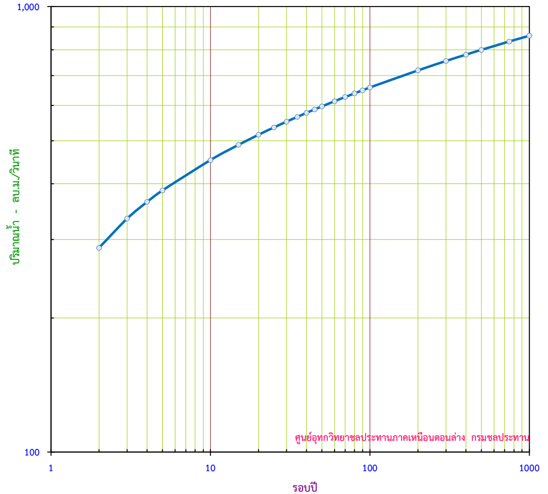
กราฟแสดง ปริมาณน้ำสูงสุดรายปี ขนาดรอบปีต่างๆ สถานี Y.42 อ.โพธิ์ประทับช้าง จ.พิจิตร
